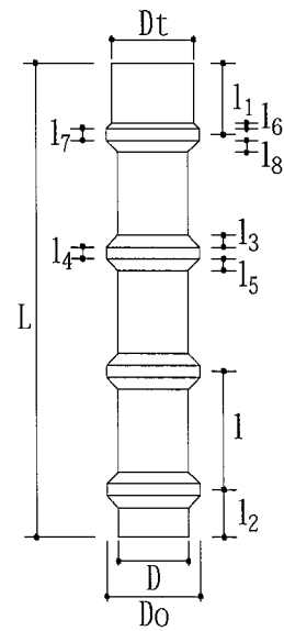
図-別-4 拡頭節ぐい (中間径タイプ)
