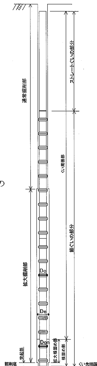
図・別-1 基礎ぐい設置概要図
